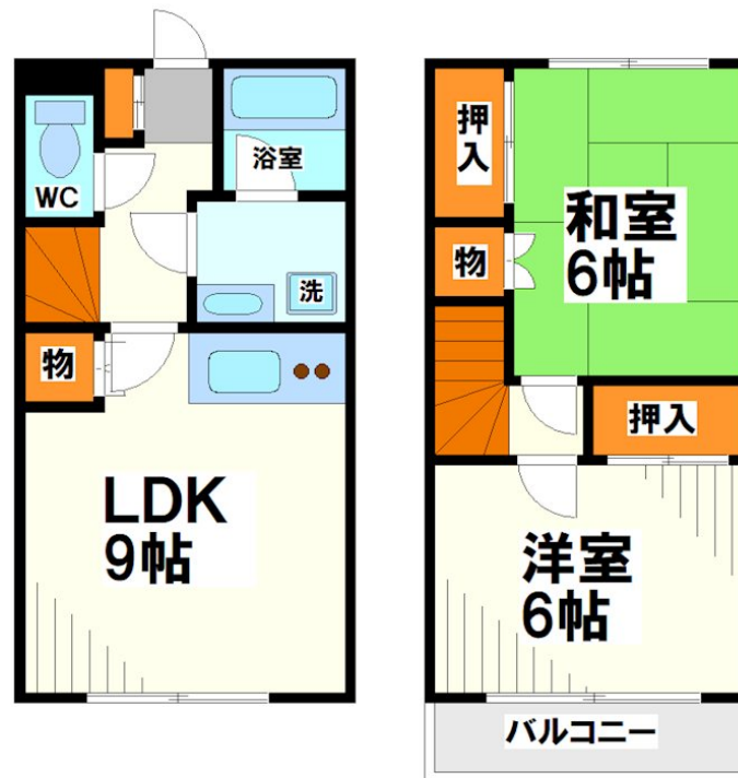
【間取り図】
